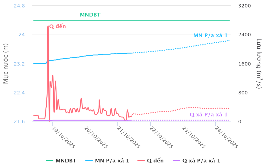
Hình 3: Phương án xả lũ hồ Dầu Tiếng
