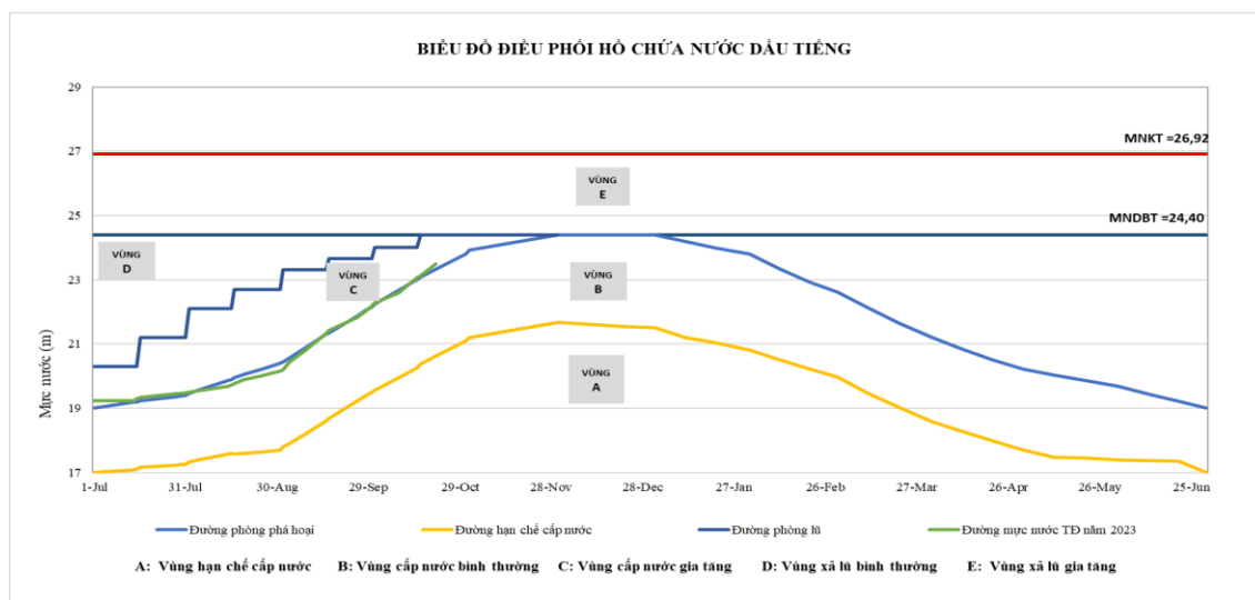
Hình 1: Biểu đồ điều phối hồ Dầu Tiếng
